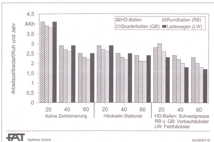
Abb. 6. Der arbeitswirtschaftliche Vergleich für Stroh ernten, aufbereiten und einstreuen zeigt, dass die Vorteile einer Strohaufbereitung überwiegen. Die Form der Strohaufbereitung hat im Boxenlaufstall allerdings einen relativ geringen Einfluss auf den Arbeitszeitbedarf.
