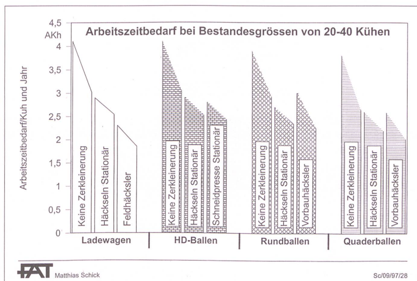
Abb. 7. Der Vergleich verschiedener Ernte- und Aufbereitungsverfahren macht deutlich, dass – bei allen Verfahren ohne vorgeschaltete Strohaufbereitung – die zunehmende Bestandesgrösse einen starken Einfluss auf den Arbeitszeitbedarf hat.
