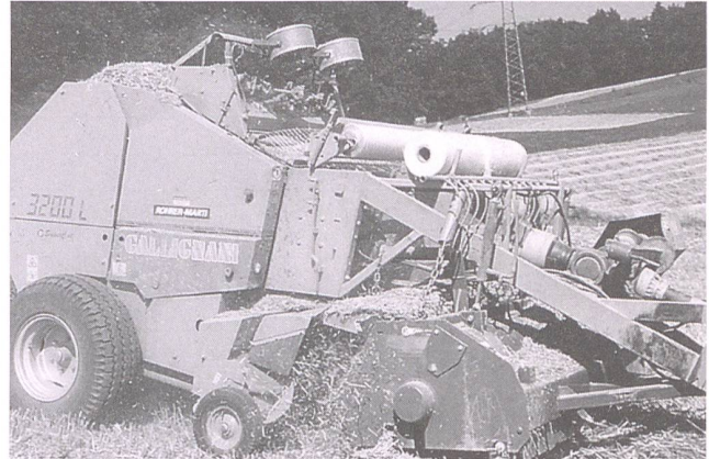
Abb. 2. Vorbauhäcksler an Grossballenpressen zerkleinern das Stroh bereits auf dem Feld. Die Staubbelastung und die Brandgefahr des Strohmahlens entfallen. Der Zerkleinerungsgrad hängt von der Einstellung und der Fahrgeschwindigkeit ab.
