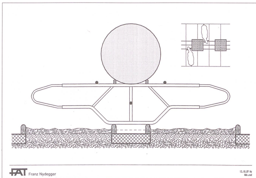
Abb. 10. Grossballen können unter Einhaltung des Platzbedarfes der Kuh über den Boxentrennbügeln gelagert werden. Das Einbringen der Ballen erfordert jedoch Einfahrmöglichkeiten in die Laufgänge.
