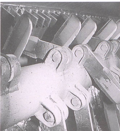
Abb. 3. Der Vorbauhäcksler (links) weist eine horizontale Welle mit beweglichen Schlegelmessern auf. Ein bis zwei Gegenschneiden sind am Gehäuse montiert. Die Schneidpresse (rechts) dagegen verfügt über sechs stehende Messer. Ein Hydraulikzylinder drückt den Strohballen durch diese Messer.
