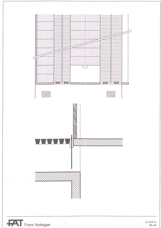
Abb. 9. Auch Kanäle unter Spalten- oder Lochböden können Langstroh verkraften, wenn sie direkt in die Güllegrube münden. Der Abschluss muss allerdings mit einem Schieber und nicht mit einem Siphon erfolgen.
