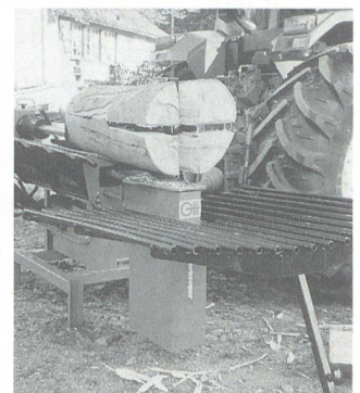
Ott: Spaltgigant Spalkkraft 30 t; Spalllänge 1250 mm; Gewicht 770 kg; fernbe- diente hydraulische Verstellung des Spaltkreuzes; Doppelpumpe; aufklappbarer Spalttisch, hydrauli- scher Ladearm; Zapfwellenantrieb; Preis: Fr. 10 300.-.
