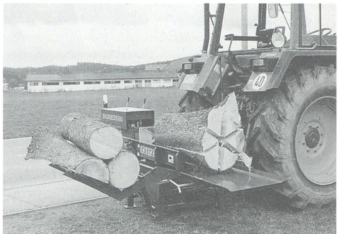
EMS: Kretzer Typ SK 900/18 Spalkkraft 18 t, Spalllänge 1150 mm, hydraulische Hubschwinge 500 kg, Gewicht 600 kg, Leistung ca. 5-8 Ster/h; Preis Fr. 7250.-.
