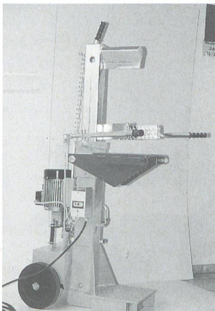
GEBA: Hydrospalter «Formula» Spalkkraft 8 t; werkzeuglose Montage und Demontage des Meterbeils, dadurch rasches Umstellen von Kurz- auf Meterholz; Zyklus Vorlauf: 9 sec, Rücklauf 3 sec.; Max. Spalllänge 1100 mm; Elektromotor 3 PS/400 V; Preis Fr. 2980.-.
