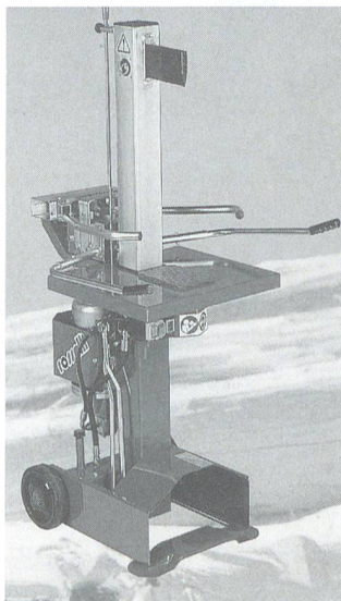
Fankhauser: Rosselli GT 1110 Spalkkraft 6 t; Spalllänge 550 mm; vorgesehen für den Betrieb mit 230 V Wechselstrom (gleiches Modell auch für 400 V erhältlich); das gleiche Modell kann auch mit 9 t Spalkkraft und wegschwenkbarem Arbeitstisch (Spalllänge bis 1100 mm) ausgerüstet werden. Gewicht 127 kg; Preis Fr. 2040.-.
