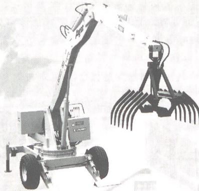
Hydrauliklader
