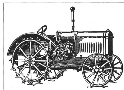
IHC-Traktor 10-20, Jahrgang 1926, mit Riemenscheibe und Heckzapfwelle.
