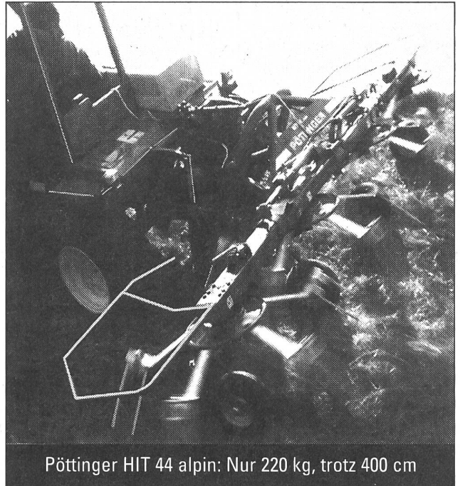
Pöttinger Ernteboss: Tieflader mit Querförderband
