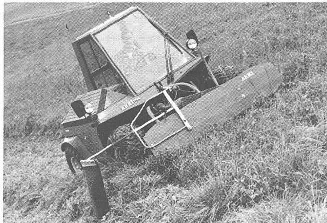
Der allerneueste Geräteträger AEBI-Terratrak TT60. Mit vier Lenkungsarten, einem total neuen Kühlerkonzept, hydrostatischem Antrieb und einem multifunktionalen Fahrhebel, mit dem man alles Wichtige im Griff hat.
