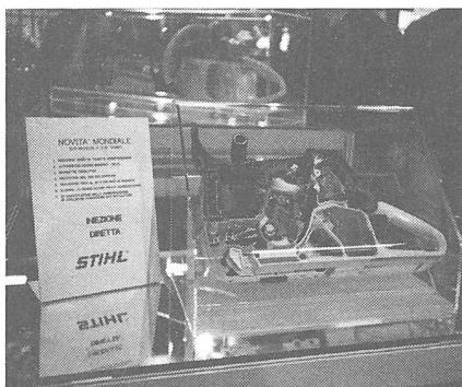
Eine Neuheit: Motorsäge mit elektronisch geregeltem Einspritzmotor zur Minimierung von Treibstoffverbrauch und Schadstoffausstoss.
