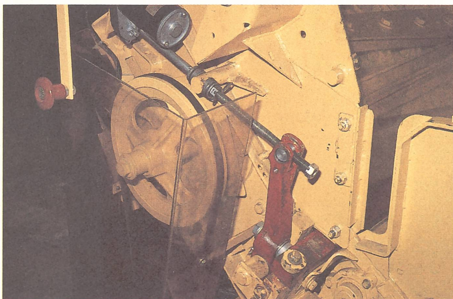
Elektronisch regulierte Gegenschneide am Feldhäcksler.
