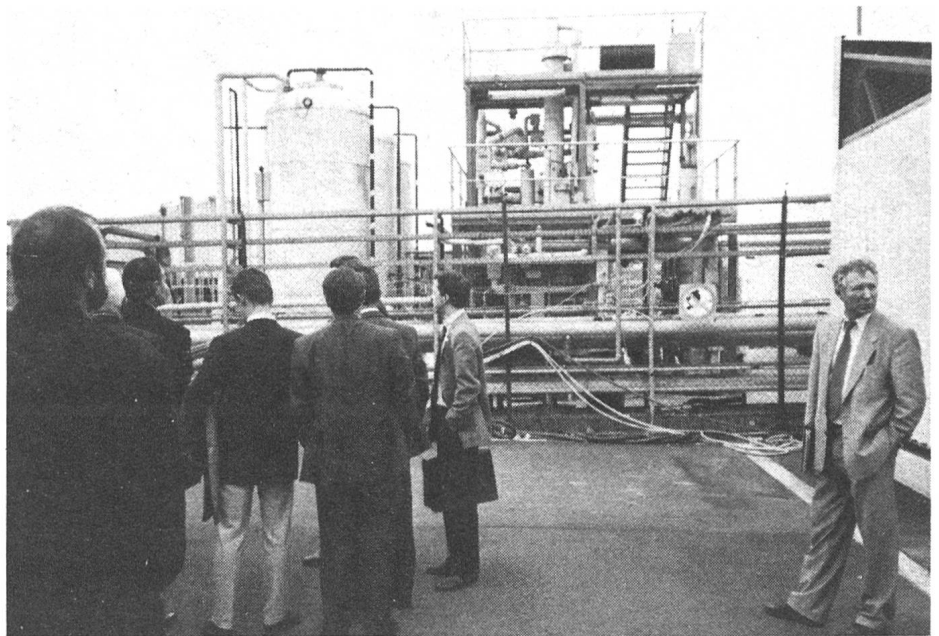
Die internationale Expertengruppe der Pilot-Umesterungsanlage auf dem Areal des Forschungszentrums der Erdölfirma Petrofina.
