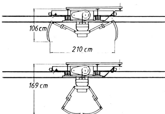
Hallenlaufkran KIWA-Elektrolift 2 TR-S, optimale Raumausnutzung und Zwei-Wagen-Trägebrücke, Hydraulikgreifer, Traglast 1250 kg, Hubgeschwindigkeit 15 und 30 m/min.
