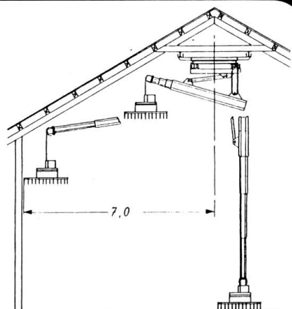
Hängedrehkran KIWA-Hydrofix 3 V-H mit dreifachem hydr. Teleskopausleger, Hydraulikgreifer an zwei getrennten Lastseilen, max. Traglast 1000 kg, Hubgeschwindigkeit 30 m/min.
