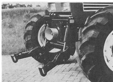
Fronthydraulik mit aufklappbaren Unterlenkern.
