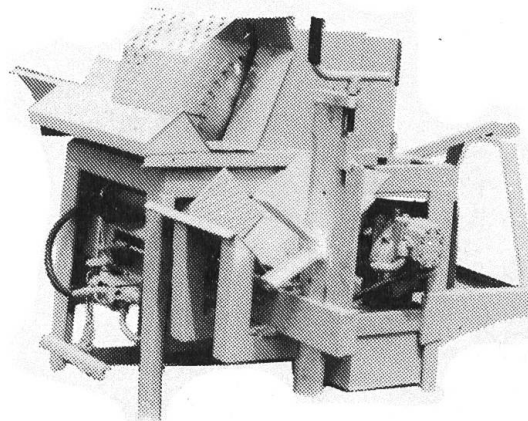
GEBA «Fräs-Spalten» fräst und spaltet das Brennholz in einem Arbeitsgang. Typ FS-Z für Zapfwellenantrieb, FS-ZE für Zapfwellenantrieb und aufgebautem 9,5 kW Elektromotor. Die grosse Neuheit!
