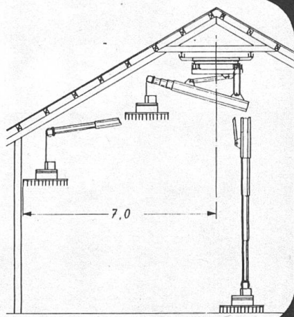
Hängedrehkran KIWA-Hydrofix 3 V-H mit dreifachem hydr. Teleskopausleger, Hydraulikgreifer an zwei getrennten Lastseilen, max. Traglast 1000 kg, Hubgeschwindigkeit 30 m/min.
