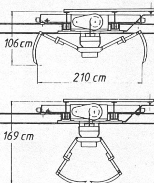
Hallenlaufkran KIWA-Elektrolift 2 TR-S, optimale Raumausnutzung und Zwei-Waben-Trägerbrücke, Hydraulikgreifer, Traglast 1250 kg, Hubgeschwindigkeit 15 und 30 m/min.
