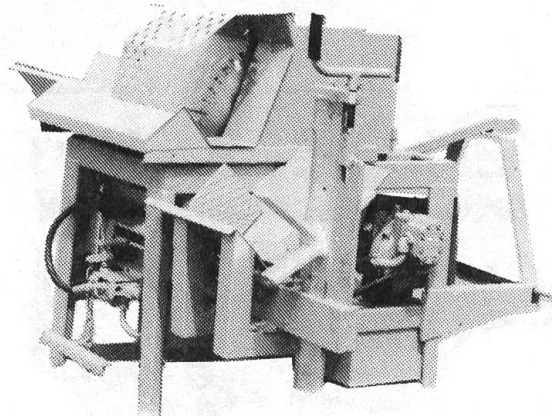
GEBA «Fräs-Spalten» fräst und spaltet das Brennholz in einem Arbeitsgang. Typ FS-Z für Zapfwellenantrieb, FS-ZE für Zapfwellenantrieb und aufgebaute 9,5 kW Elektromotor. Die grosse Neuheit!
