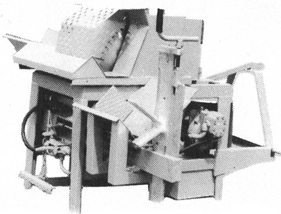
GEBA «Fräs-Spalten» fräst und spaltet das Brennholz in einem Arbeitsgang. Typ FS-Z für Zapfwellenantrieb, FS-ZE für Zapfwellenantrieb und aufgebautes 9,5 kW Elektromotor. Die grosse Neuheit!
