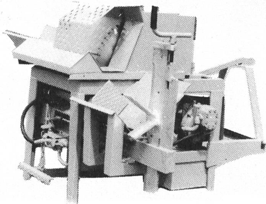
GEBA «Fräs-Spalten» fräst und spaltet das Brennholz in einem Arbeitsgang. Typ FS-Z für Zapfwellenantrieb, FS-ZE für Zapfwellenantrieb und aufgebaitem 9,5 kW Elektromotor. Die grosse Neuheit!
