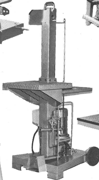
GEBA Hydrospalter bis 7 t Spalkkraft, Holzlängen bis 107 cm, mit Elektro- oder Benzinmotor.
