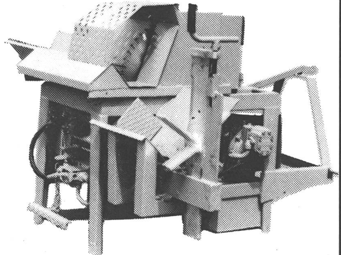
Kombi Brennholzkreissäge fräst und spaltet in einem Arbeitsgang. Die rationelle Lösung.
