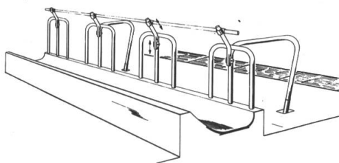
"Waldstätter", Typ "SR" mit verstellbarem Stopprohr BVET Nr. 14156
