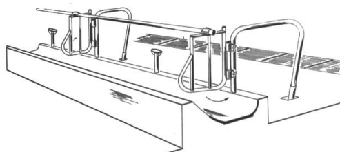
"Enorm-Plus", Typ "E" mit oder ohne Fressbügel BVET Nr. 14159
