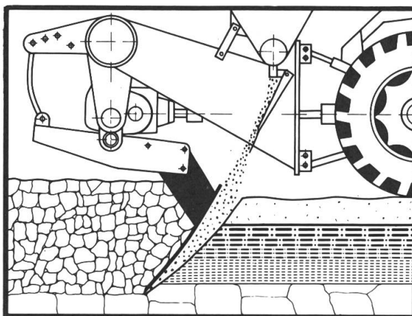
Tieflockerung mit gleichzeitiger Einarbeitung von Zusatzstoffen
