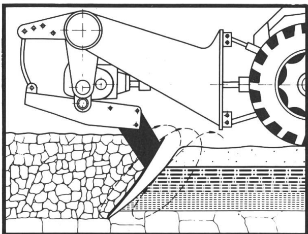
Lockerung bis 70 cm Tiefe
