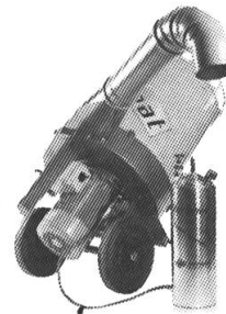
Strohmühle Vakuumat
