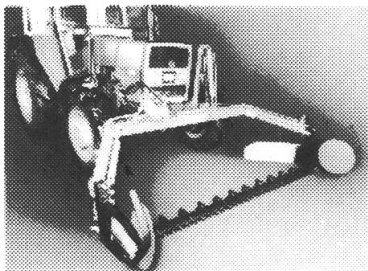
KURMANN-Frontmäherwerk mit Busatis Doppelmesserschneiderwerk 2,5 m
