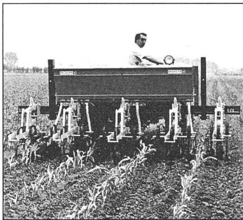
BADALINI-Hackgerät
