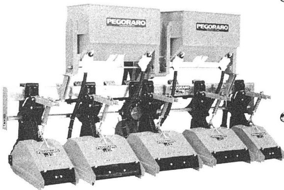
PEGORARO-Reihenfräse
