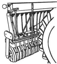
Einzelkornsämaschine Becker, neu! Coulter Scheibe und Unterschneidschar für Direktsaat in 2-jährigen Bestand
