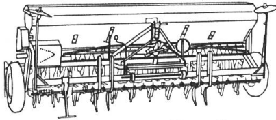
Einzelkornsämaschine Becker, neu! Coulter Scheibe und Unterschneidschar für Direktsaat in 2-jährigen Bestand
