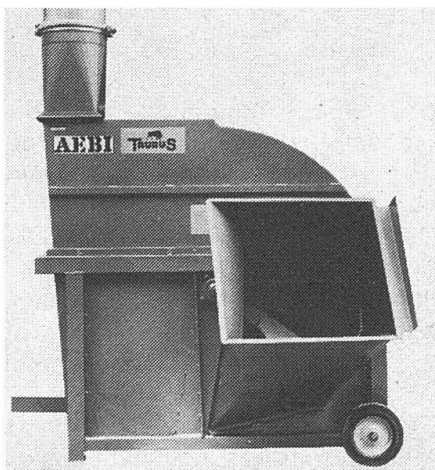
Taurus-Silierkanone.
