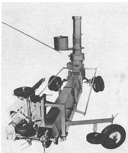
Taurus-Saugfräse.
