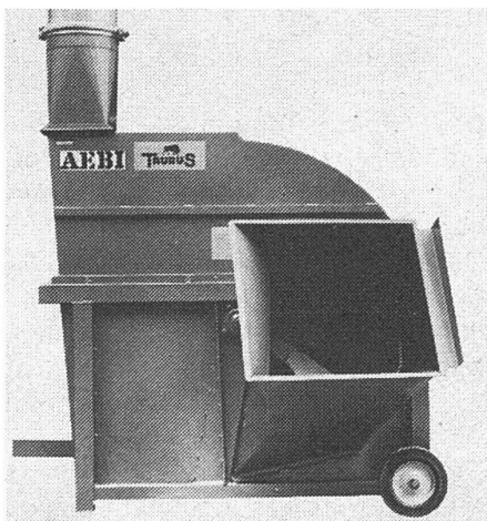
Taurus-Silierkanone.
