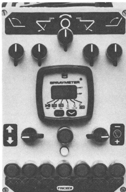
Fischer Spraymeter das elektronische Kontroll- und Steuergerät für den Kabineneinbau.
