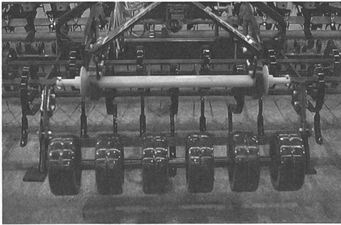
4+5: Rückverfestigung des Bodens zwischen den Radspuren.
