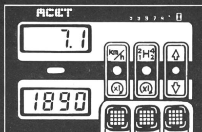
ACET Bordcomputer für computerüberwachte Wirtschaftlichkeit.
