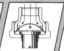
Präzisions- düsen aus Edel-Keramik für absolut prä- zise Verteilung.
