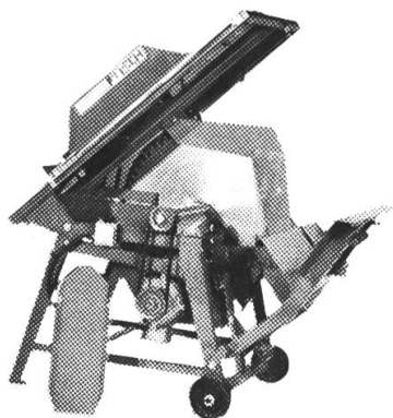
Mit Wipp-Tisch, El.-Motor und Keilriemenantrieb
