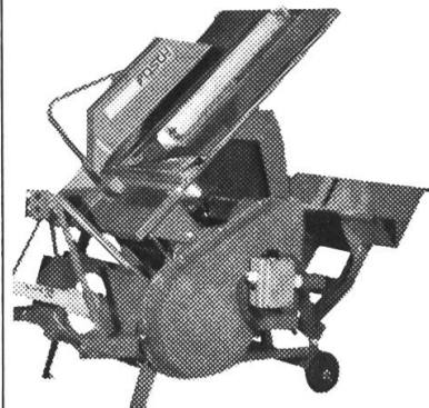
Wipp-Tisch und Antrieb kombiniert Zapfwelle/ Elektro-Motor
