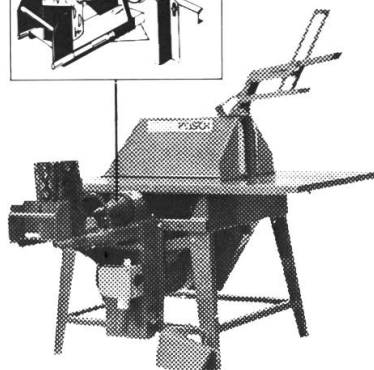
Mit Rolltisch und Brennholzspalter*)
