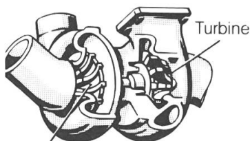
Verdichter (Lader)
