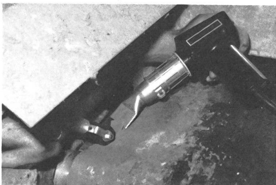
LEISTER beim Schweissen eines Randdefektes an einem PVC-beschichteten Förderband.
