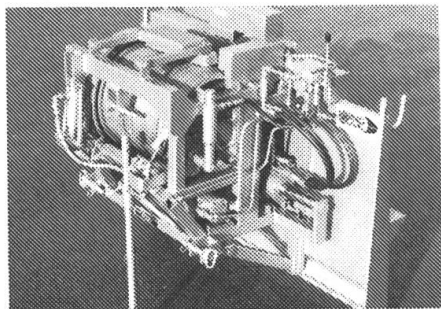
Bärtschi Seilwinde , hydr. gesteuerte Seilführung, grosse Seilaufnahme.
