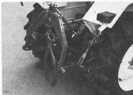
Bärtschi Holzschleppzange für Traktorhydraulik und Seilzug. Kat. I und II.
