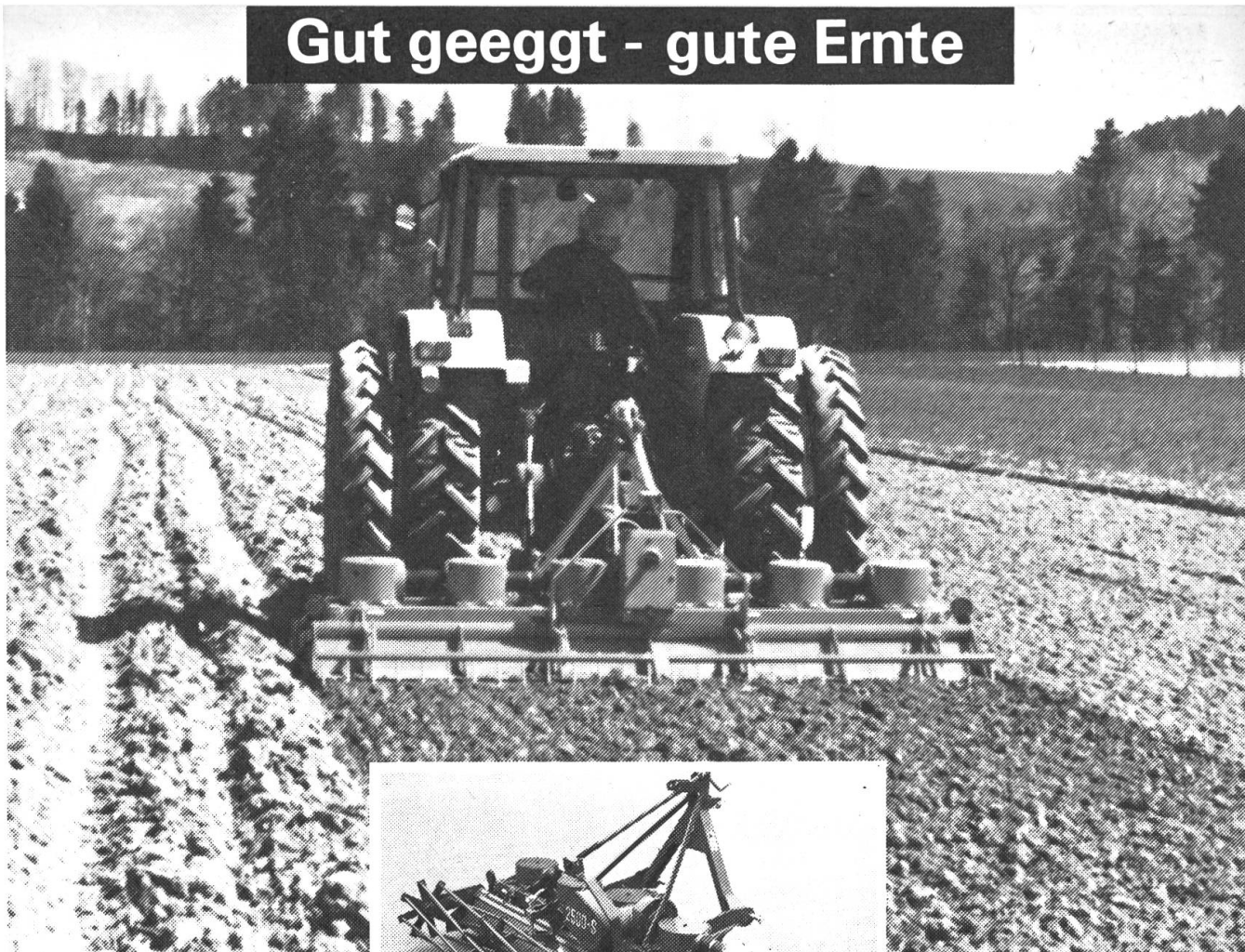
Schweizer Kreiselegge TORONADO
