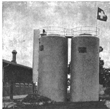
Biogasanlage auf Landwirtschaftsbe- trieb mit 100 GVE (Grossvieheinheiten)
