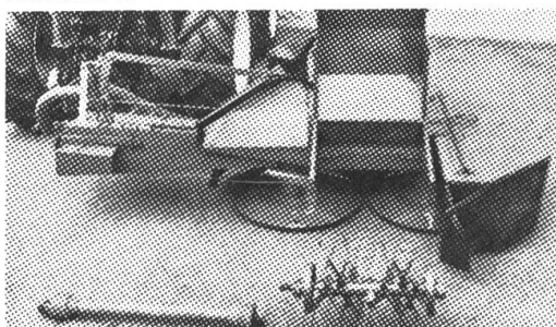
Fahr Kreiselmäher KM 22 CR mit an- und abbaubarem Fingerrotor.
