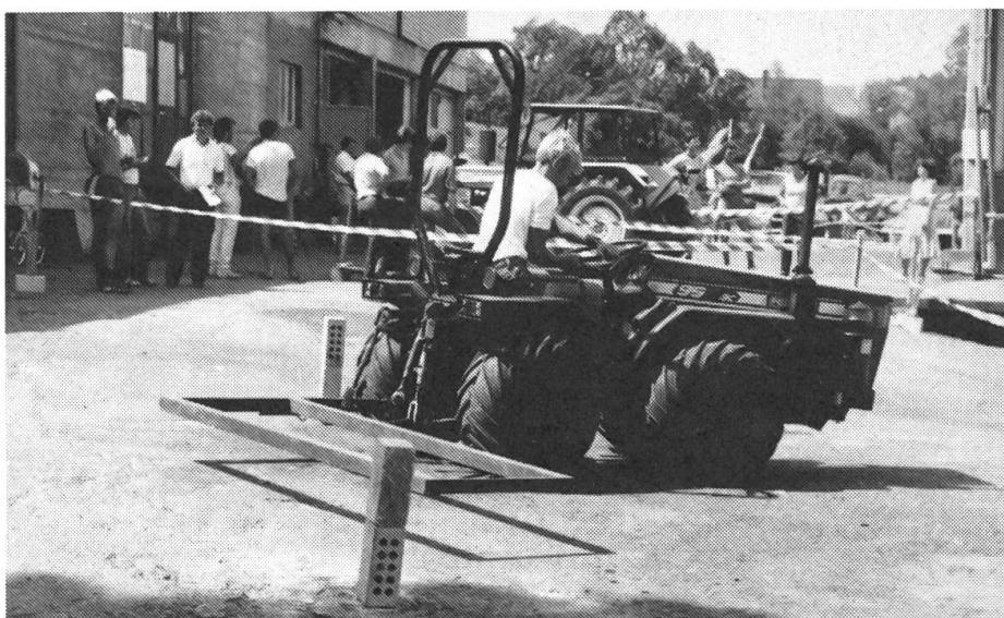
Abb. 2: Fahren mit einem Knicklenker-Traktor in einem Parcours. Vorsicht, beim Lenken bewegt sich auch der Anbaurahmen.
