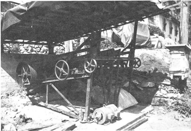
Abb. 1: Diese Bergstation steht in Loco, Val Orsenone TI. Sie musste auf Elektrobetrieb umgebaut werden, damit Lärmemissionen vermieden werden können.
