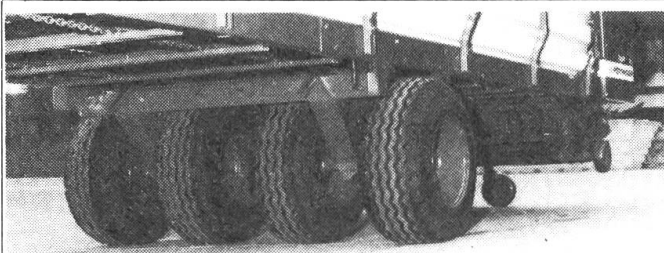
Die optimale Last- und Bodendruckverteilung
