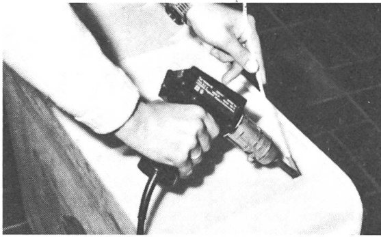
LEISTER beim Reparaturschweissen von einem Polyäthylen-Behälter
