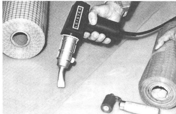
LEISTER beim Schweissen eines Randdefektes an einem PVC-beschichteten Förderband.
