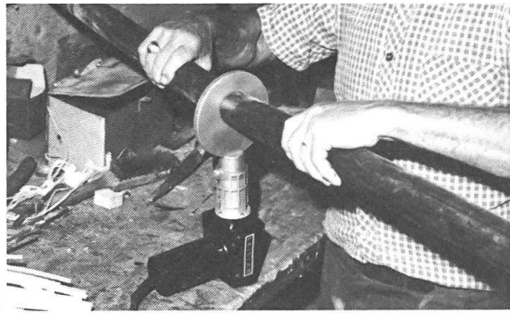
LEISTER beim Stumpfschweissen von Polyäthylen-Rohren.
