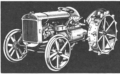
Jahrgang 1933 Erster Ferguson-Traktor mit 3-Punkt-Hydraulik, 28 PS
