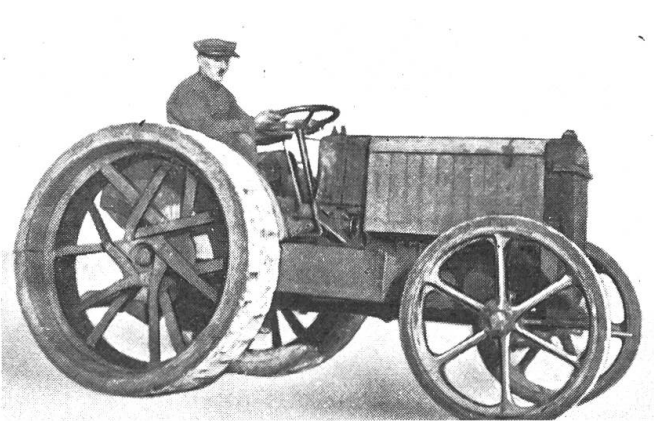
Austin-Traktor (1920), importiert aus Frankreich durch Firma Blatter in Zürich, 4-Zylinder-Benzinmotor (Photo H. Beglinger †).
