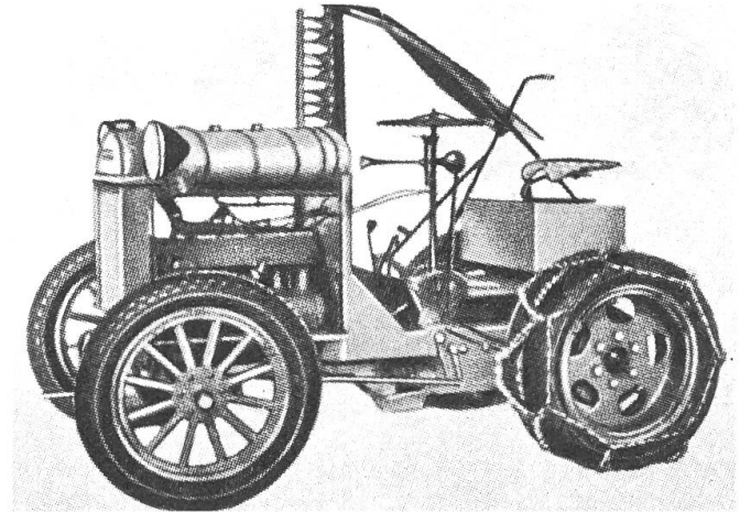
Bühler-Traktor , (1929) 1. Modell mit Ford-Motor T, 4 Zyl., (White-Sirit), hergestellt von Fritz Bühler, Frauenfeld (Photo H. Beglinger †).
