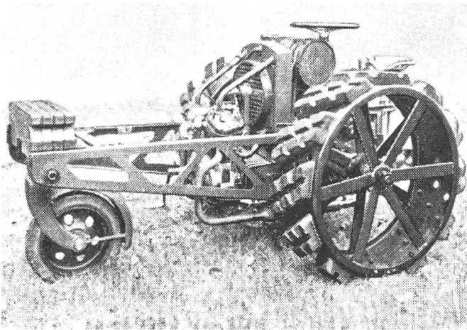
Mafag-Traktor , eine Weiterentwicklung des Universal, hergestellt durch die Maschinenfabrik Brugg (später Müller AG). (1929) – Photo H. Beglinger †.
