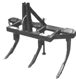
ZAUGG-Tiefenlockerer
