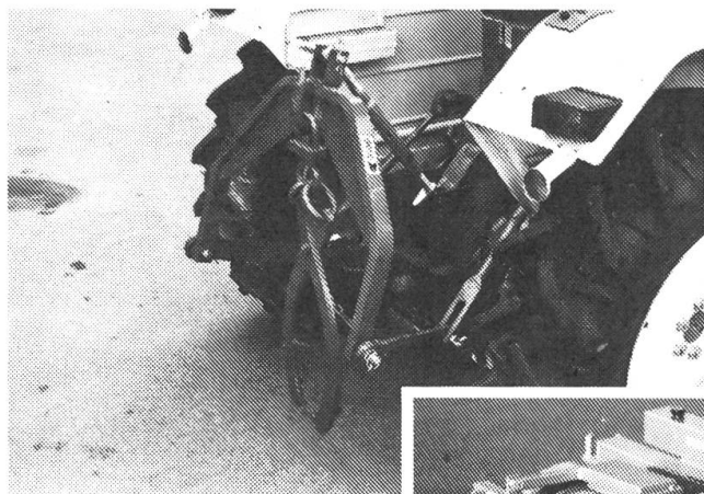
Holzschleppzange Bärtschi
