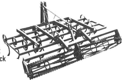
ZAUGG-Federzinken-Egge
