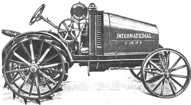
Traktor International 8/16 (1919), importiert durch die IHC, Zürich. 4-Zyl.-Petrolmotor mit Kettenantrieb.
