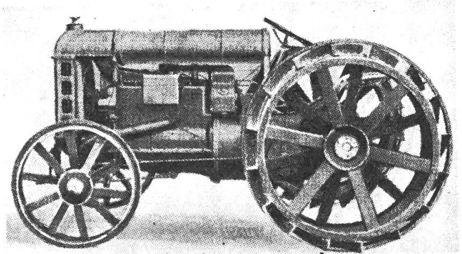
Traktor Fordson (1919), importiert durch die damalige Generalvertretung Garage Addor, Lausanne. 4 Zyl. 22 PS.
