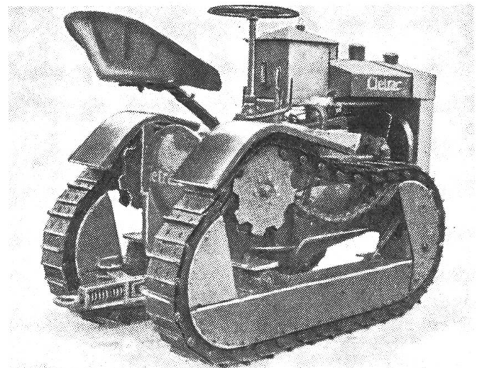
Raupentraktor Cletrac, Mod. F. (1919), importiert durch Fritz Marti AG, Bern. Benzin/Petrol-Motor. 16 PS.
