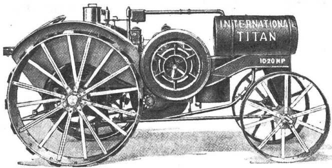
Traktor Titan (1917), importiert durch die International Harvester Company, Zürich. 2-Zyl.-Petrolmotor mit Kettenantrieb.
