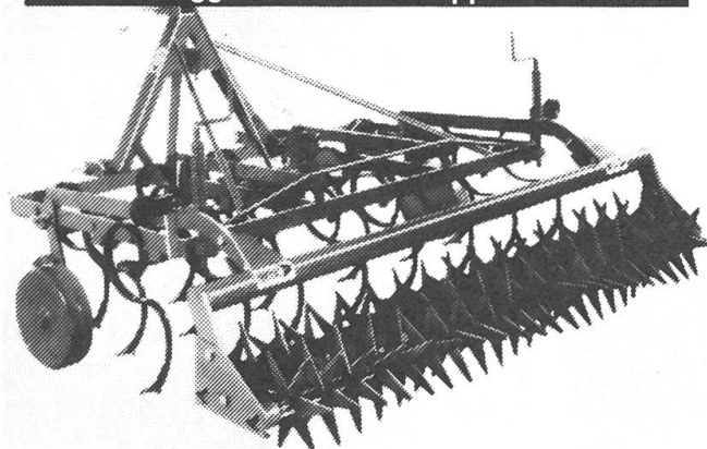
Federzahnegge Bärtschi mit Doppelsternkrümmer
