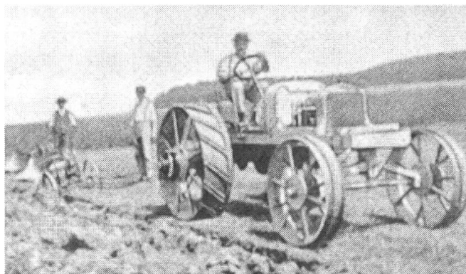
Aus verschiedenen Lastwagenteilen hergestellter Traktor mit Martini-Motor (ca. 1919).
