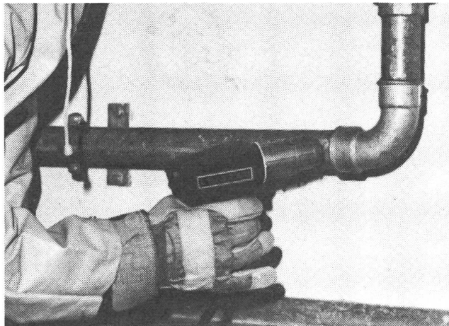
Auftauen von Wasser- und Diesel-Leitungen am Traktor im Winter mit dem kräftigen Heissluftstrahl des Leister-Ghibli. Warmluftzufuhr in den Ansaugkanal des Vergasers bedeutet Starthilfe.
