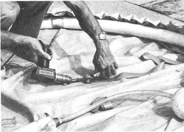
Reparaturschweissung an einer wassergefüllten Silopresse. Blachen und Traktorplanen bestehen meistens aus gut schweisssbaren Polyätylen- oder PVC-Folien.
