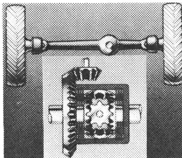
Der Allrad-Antrieb wird während der Fahrt über einen Kippschalter zuge- schaltet. Die automatische Differential- sperre des Frontantriebs, eine Zusatz- ausrüstung, verhindert zuverlässig Rad- schlupf.
