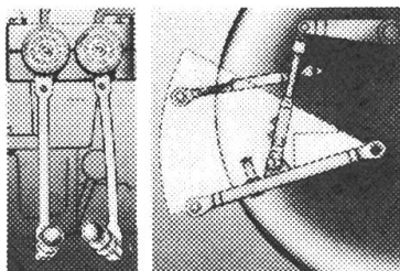
Große Ölflußmenge und 190 bar Druck erlauben große Hubleistungen an der 3- Punkt-Hydraulik. Auch Geräte-Hydrau- likzylinder werden zuverlässig mit Öl versorgt.
