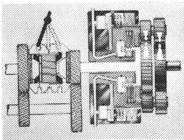
Konische Synchronringe erlauben mühe- losen, präzisen Gangwechsel während der Fahrt.
