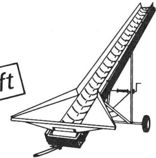
Gummi-Förderbänder Gurt flach, muldenförmig oder Wellenkante
