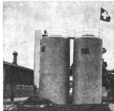
Biogasanlage auf Landwirtschaftsbe- trieb mit 100 GVE (Grossvieheinheiten)
