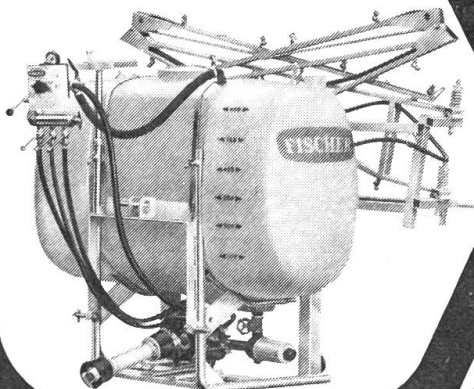
Aufsattelspritze FISCHER-AGRIFIX
