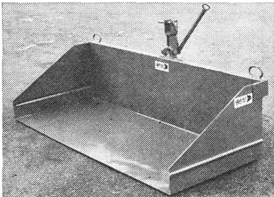
Bärtschi Mehrzweck-Ladeschaufel mit Rollen-Kippvorrichtung, leicht ausklinkbar, sicher, keine Pneubeschädigungen. 3 Grössen, auf Wunsch mit Rückwand-Erhöhung. NEU! Verschleissmesser aus Spezialstahl
